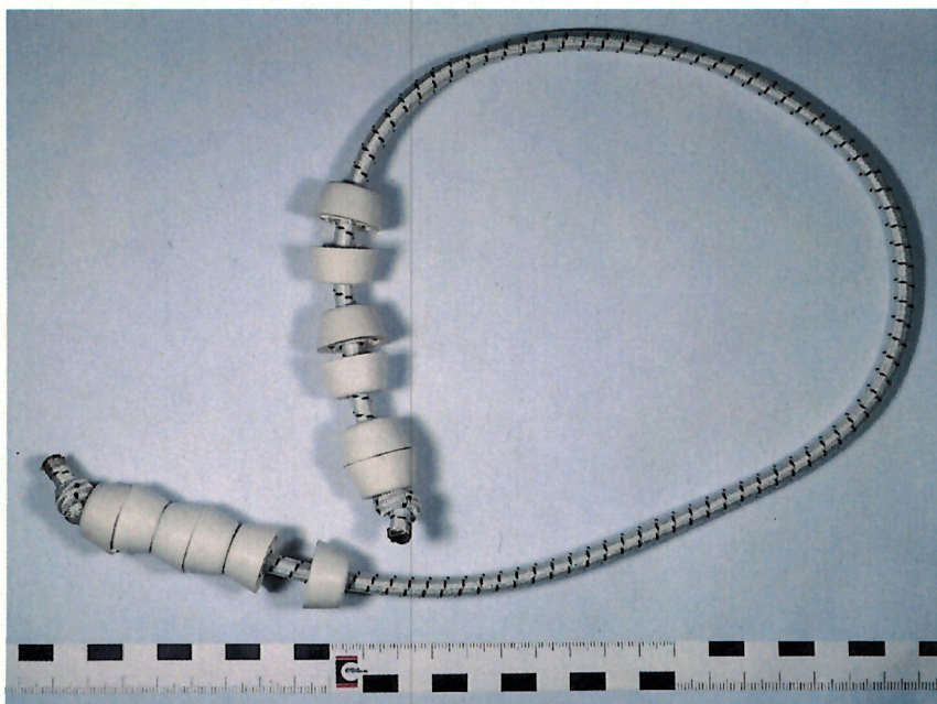
Abbildung 2 – Ausführung 2 „Kegelstumpf“
